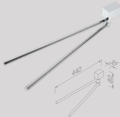
Handdoekrek 2-armig Towel rail with 2 arms 917505-02
