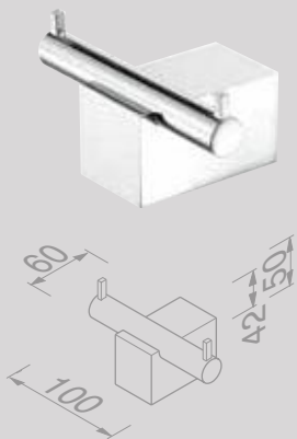
Handdoekhaak dubbel Towel hook double 917515-02
