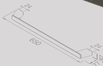
Handdoekrek 60 cm Towel rail 60 cm
