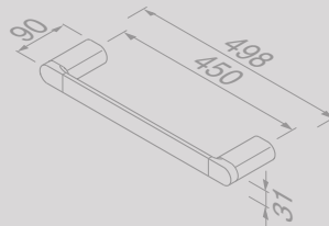
Handdoekrek 45 cm Towel rail 45 cm
