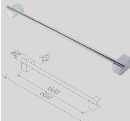
Handdoekrek 60 cm Towel rail 60 cm 917507-02
