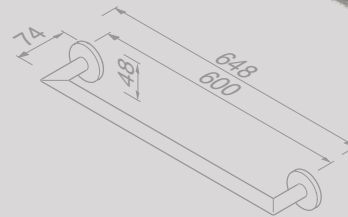
Handdoekrek 60 cm Towel rail 60 cm
